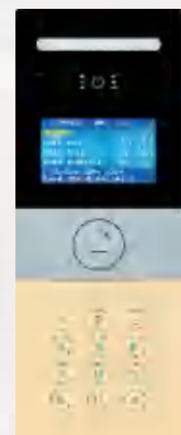
S77-4X1 4.3寸轻触按键数字主机 外观尺寸: 365×140×50mm 安装尺寸: 348×130×40mm
