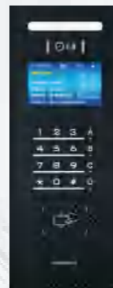
○ S88-4X9 4.3寸触摸按键人脸识别主机 外观尺寸: 380×148×50mm 安装尺寸: 345×130×40mm
