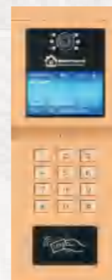
S76-1X1 4.3寸轻触按键数字主机 外观尺寸: 360×140×50mm 安装尺寸: 345×130×40mm
