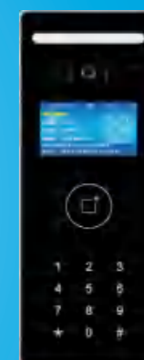
S88-5X1 4.3寸触摸按键数字主机 外观尺寸: 360×140×50mm 安装尺寸: 345×130×40mm
